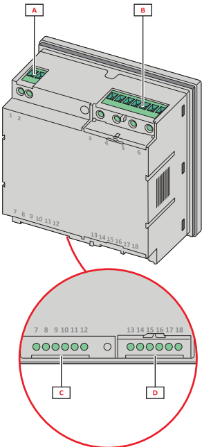
Fig. 2 Back
